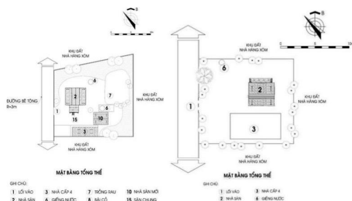
Hình 2.1 và Hình 2.2: Bố cục mặt bằng tổng thể nhà ở người Chăm H'roi (Thôn Hà Rai, Xã Xuân Lãnh - Huyện Đồng Xuân - Tỉnh Phú Yên) trước và sau tái định cư. Nguồn: Tác giả [1]
