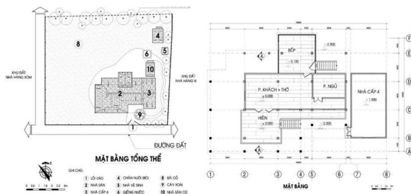
Hình 2.6 và 2.7. Mặt bằng tổng thể và mặt bằng nhà người Chăm H'roi, trường thôn Tân Hiệp (Thôn Tân Hiệp, Xã Sơn Hội - Huyện Sơn Hòa - Tỉnh Phú Yên) Nguồn: Tác giả
