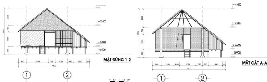
Hình 2.11. Mặt đứng chính và mặt cắt nhà dạng mái tranh phân tre truyền thống người Chăm H'roi (Thôn Tân Lương, Xã Sơn Hội - Huyện Sơn Hòa - Tỉnh Phú Yên). Nguồn: Tác giả
